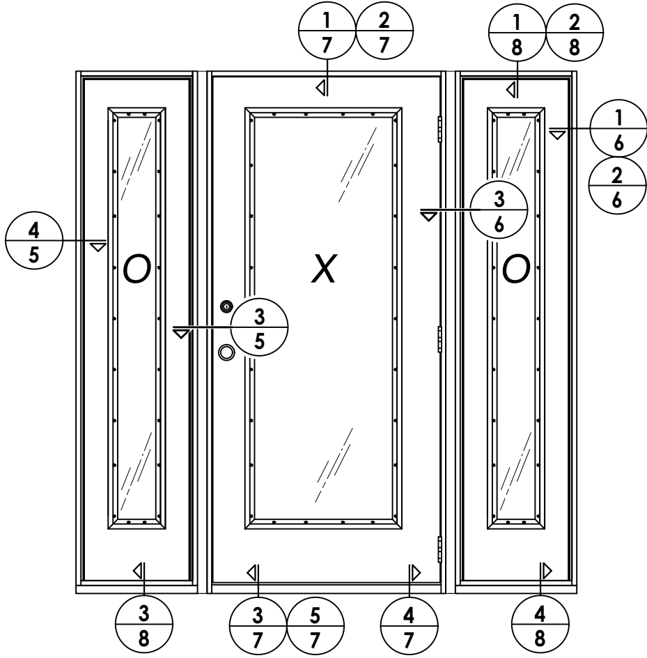
ELEVATION (OXO)
